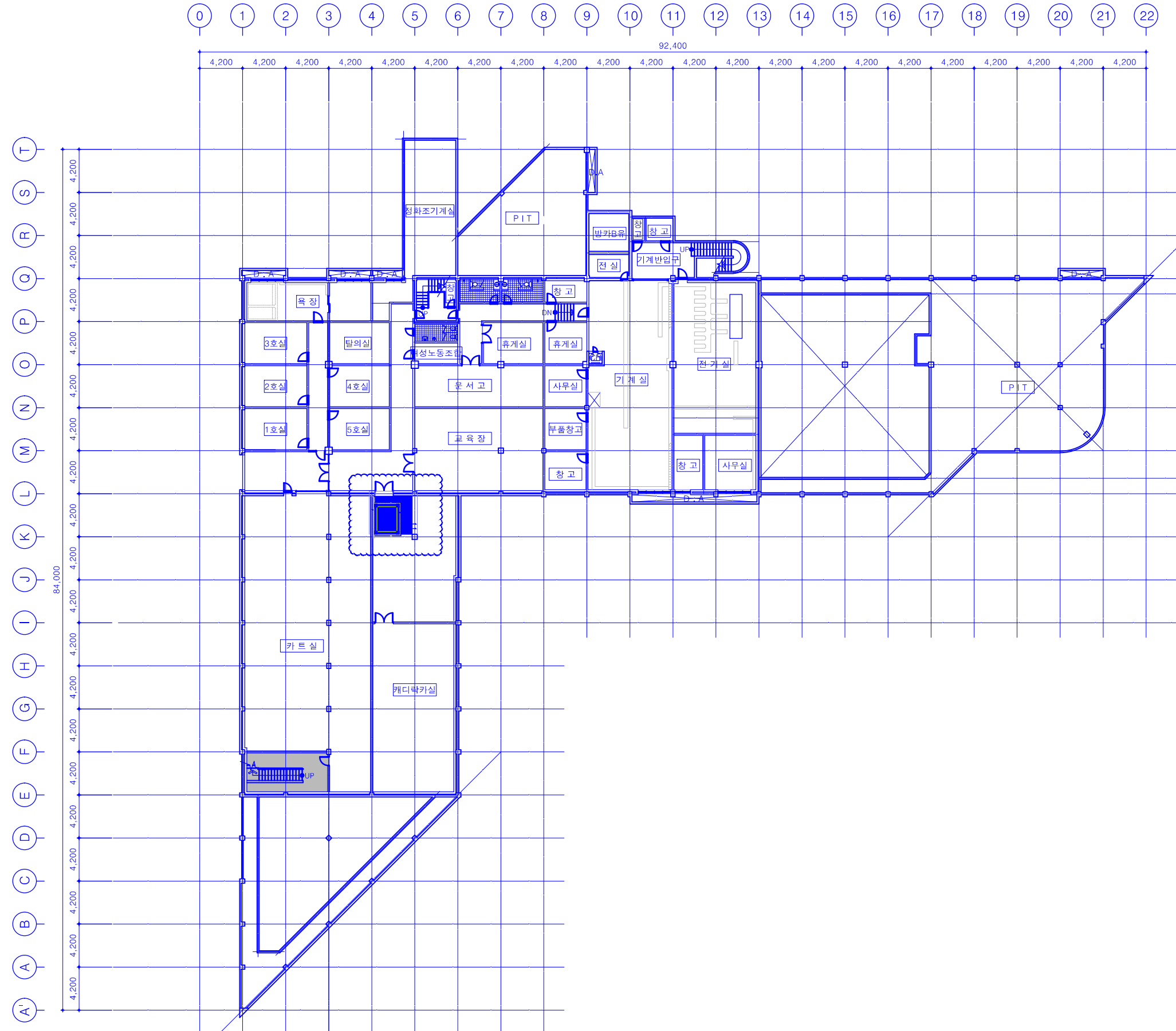
1 A 202 지하1층 평면도 SCALE : 1/200
